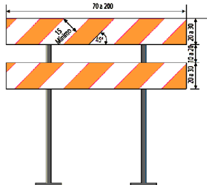
BARRERA SIMPLE TIPO II
